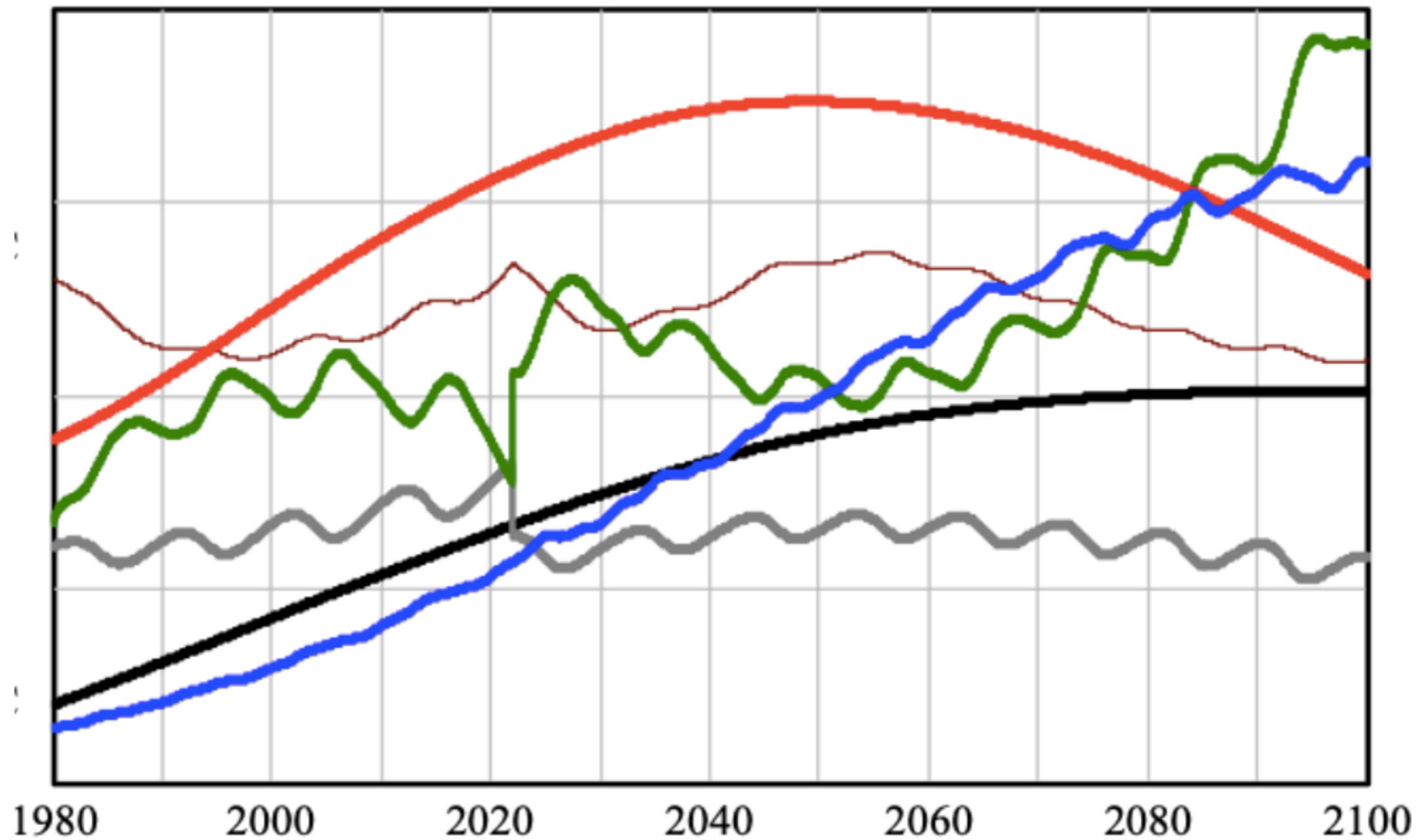
FIGURE 1. TENDANCES GLOBALES DANS LE SCÉNARIO DU "PAS DE GÉANT" DU MODÈLE EARTH4ALL – MONDE DE 1980 À 2100.
