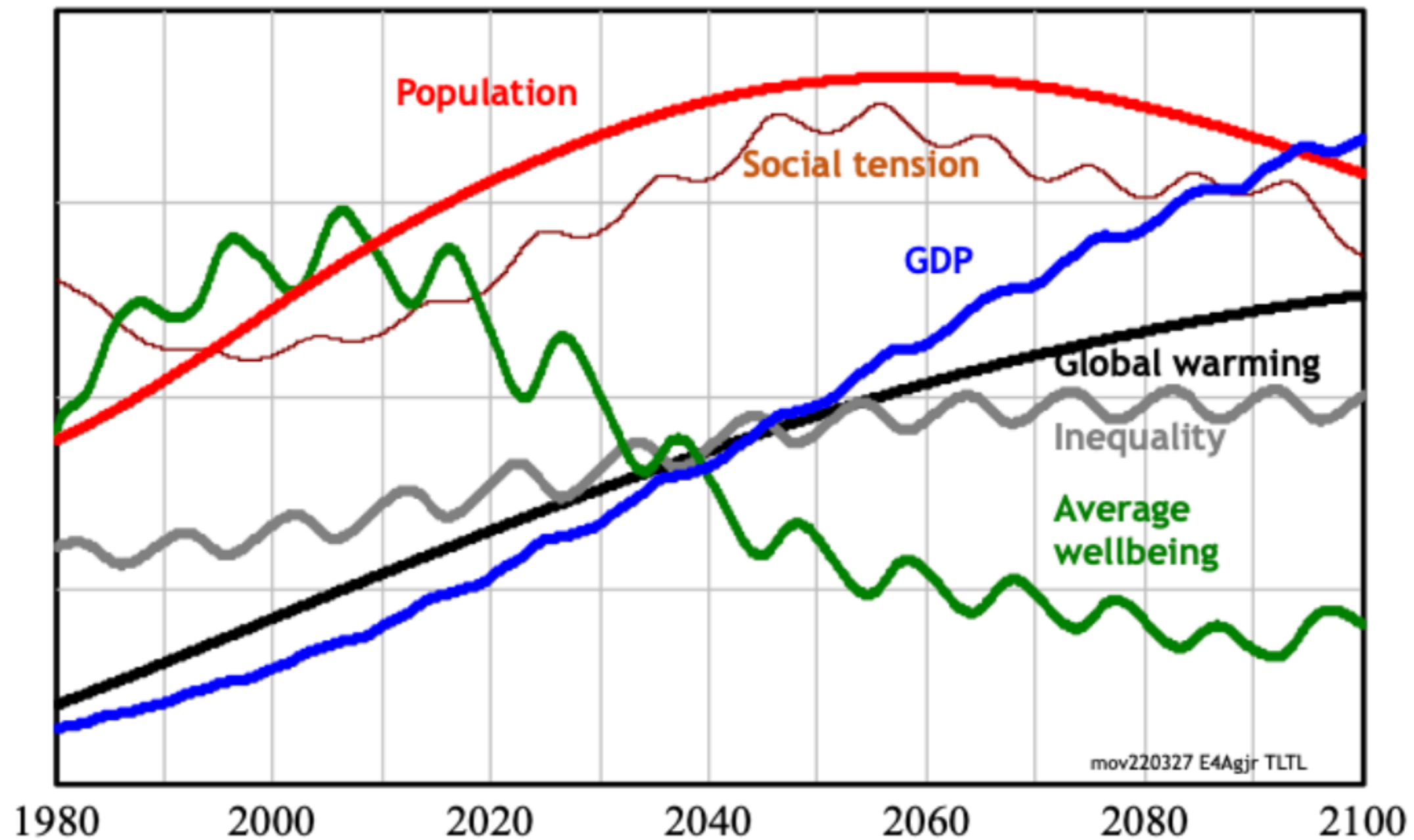
FIGURE 1. TENDANCES GLOBALES DANS LE SCÉNARIO "TROP PEU, TROP TARD" DU MODÈLE EARTH4ALL – MONDE DE 1980 À 2100.
